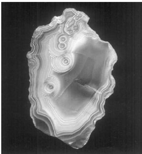
Синарский полицентричный агат
