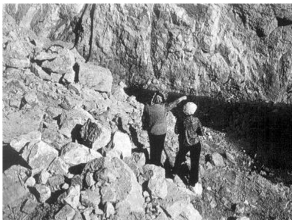
Медвежское месторождение переливта
